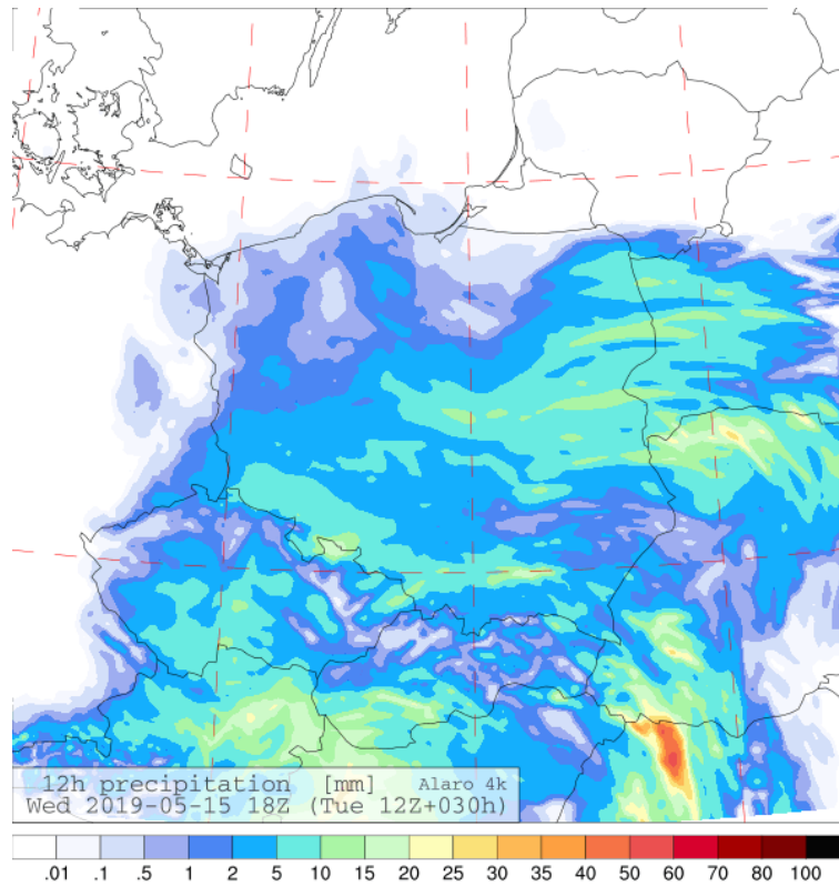
Rys. 3 Prognoza 12-godzinnej sumy opadów, środa 15.05
