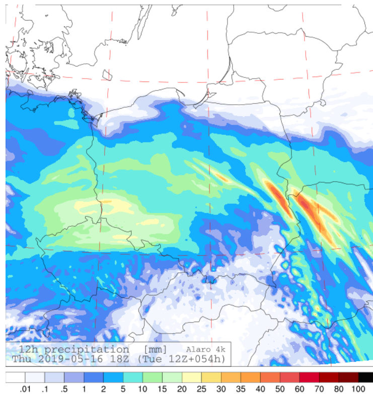
Rys. 4 Prognoza 12-godzinnej sumy opadów, czwartek 16.05
