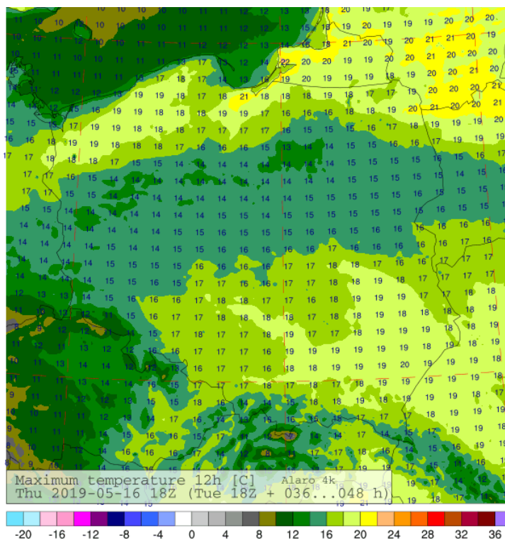
Rys. 2 Prognoza temperatury maksymalnej, czwartek 16.05
