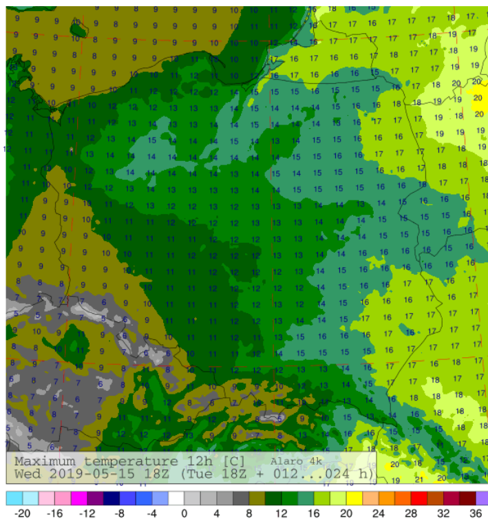
Rys.1 Prognoza temperatury maksymalnej, środa 15.05
